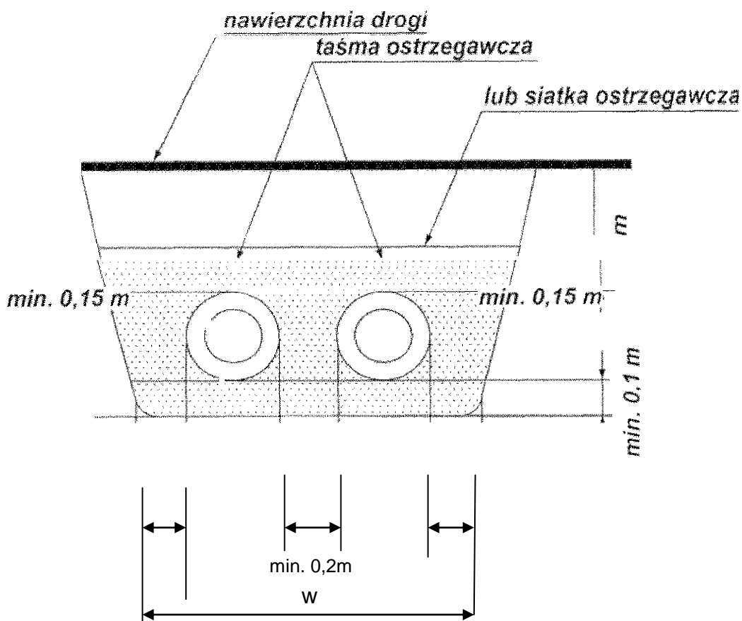
Rysunek. Przekrój i podstawowe wymagane wymiary wykopu dla rur preizolowanych
